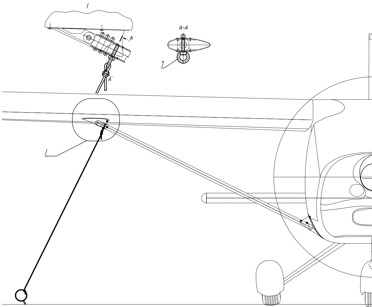
Fig. 25. Tie-down ring
